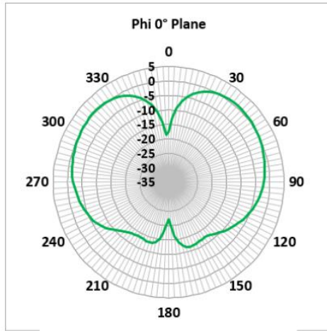
617 MHz (FTRA6171M5Px)
