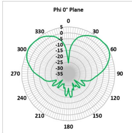
2700 MHz (FTRA6171M5Px)
