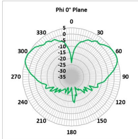
5470 MHz (FTRA6171M5Px)
