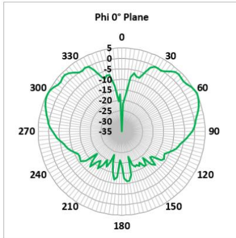
3800 MHz (FTRA6171M5Px)
