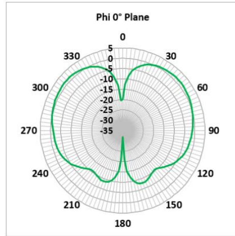
698 MHz (FTRA6171M5Px)
