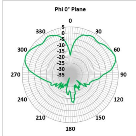
5150 MHz (FTRA6171M5Px)
