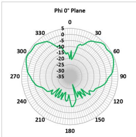
4200 MHz (FTRA6171M5Px)
