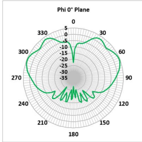
2310 MHz (FTRA6171M5Px)
