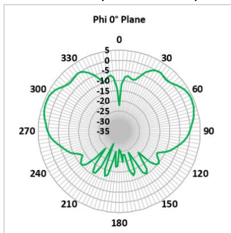
2170 MHz (FTRA6171M5Px)
