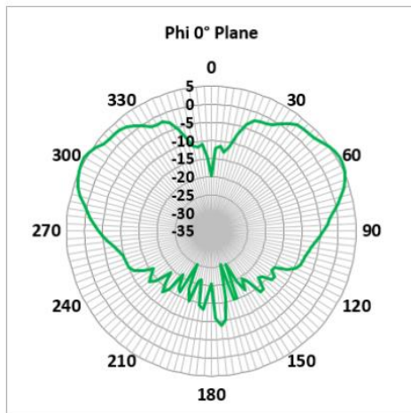
3300 MHz (FTRA6171M5Px)
