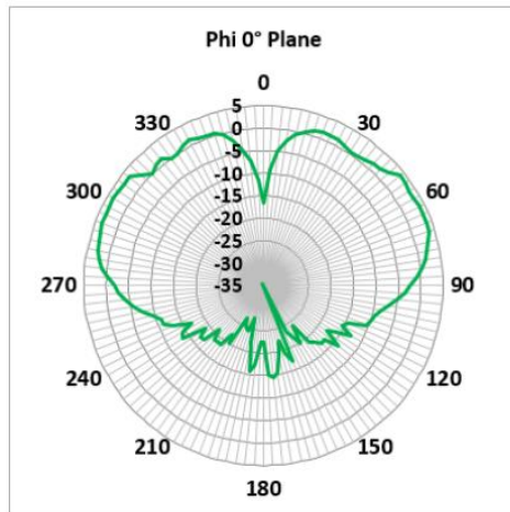
5925 MHz (FTRA6171M5Px)
