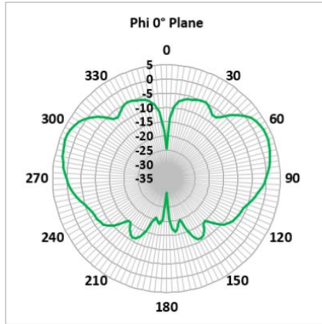
1427 MHz (FTRA6171M5Px)
