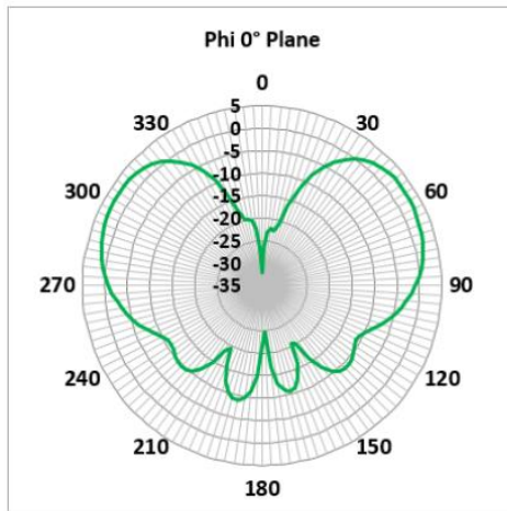
960 MHz (FTRA6171M5Px)
